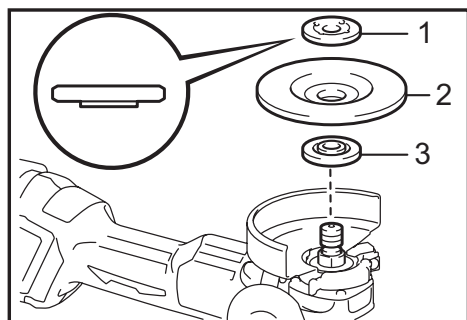
► 1. Contratuercia 2. Disco de centro hundido 3. Brida interior
