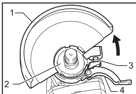
► 1. Carter de meule 2. Cage de roulement 3. Vis 4. Levier
