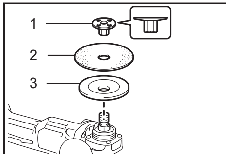
► 1. Contratuercas de lijado 2. Disco de lija 3. Plato de goma
